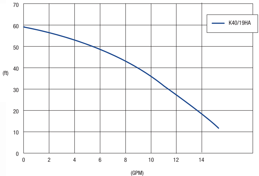
Curva de operación de las bombas
